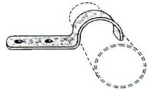
Haken f. Bretter, horizontal Art. Nr. 1240, f. 25 mm Ø
