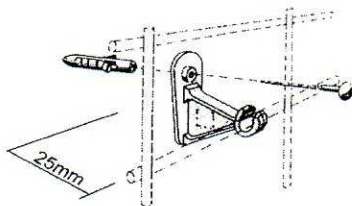
Wandhalter aus Kunststoff Art. Nr. 4001
