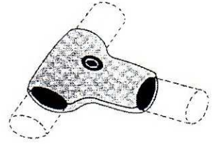
T - Verbinder m. Schraube Art. Nr. 1460, f. 25 mm Ø
