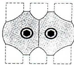
Parallelverbinder f. 3 Rohre Nr. 1270, f. 25 mm Ø
